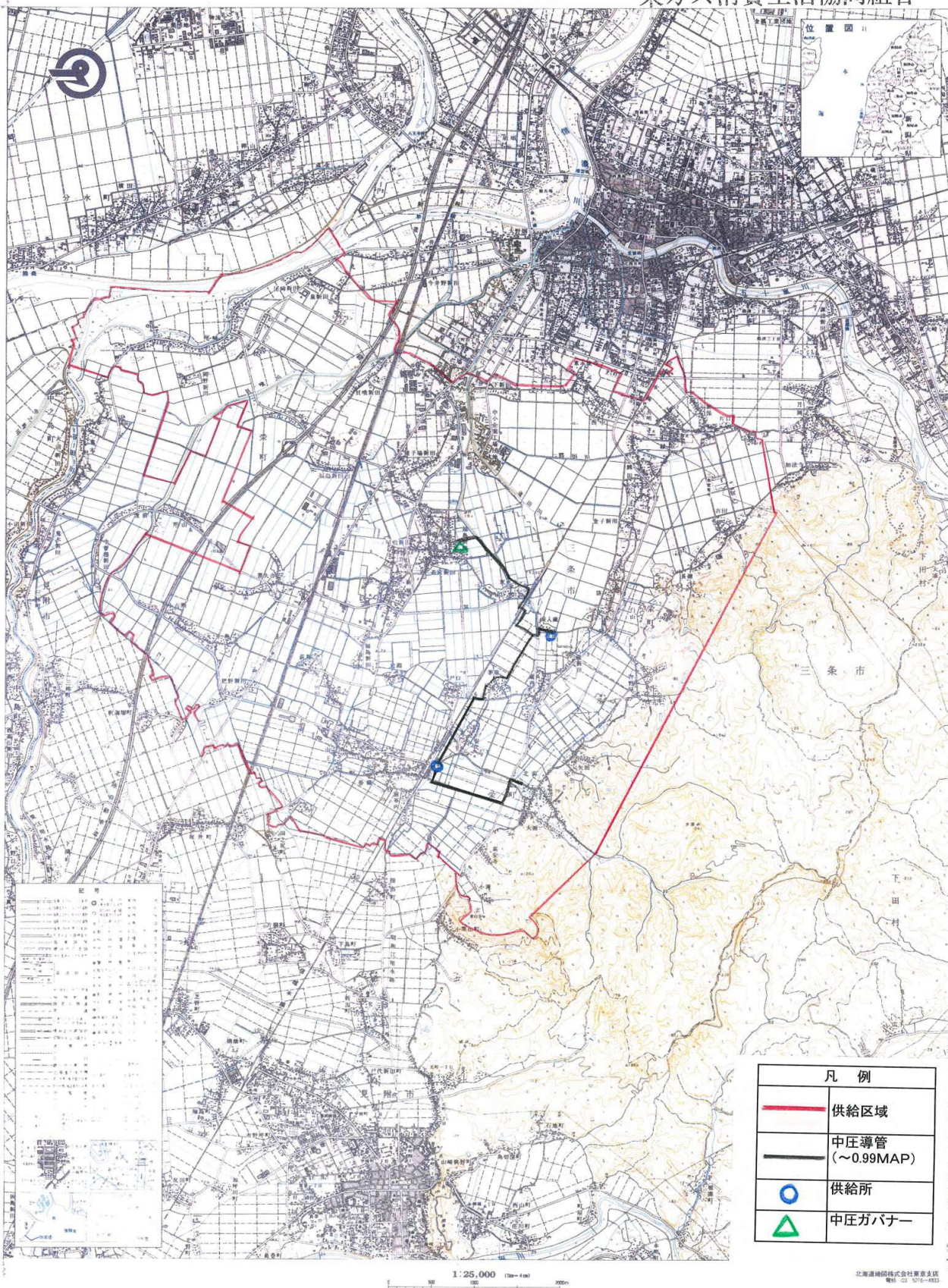
第8表 主要導管図
