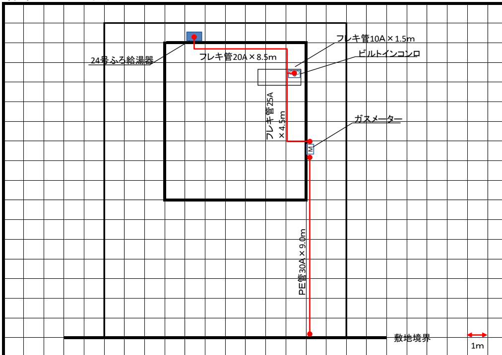
標準モデル平面図
